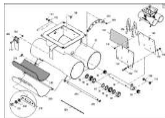
ETB-0000007721, Двойной замок 125 продольный
