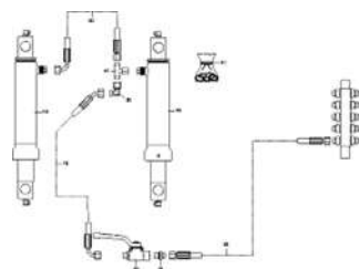
ЕТВ-0000003935, Гидравлическая схема DMC 9 м Super/XL сошники, гидравлические детали задняя навесная система
