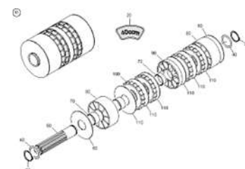
ETB-0000006978, Дозирующий ролик 40 куб. см с 8.2022
