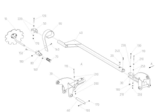
ЕТВ-6000000247, Стрела
