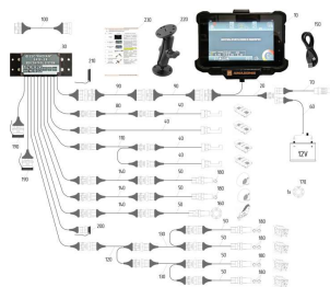
ЕТВ-6000000131 66500339 Базовый комплект электроники СКИФ-28 до 07.2025
