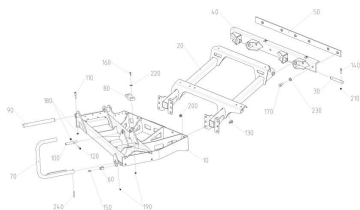
ЕТВ-6000000241, Рама правая
