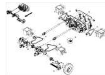
ЕТВ-0000011407, Привод задней части Primera DMC 1300 л
