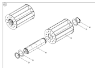
ETB-0000007929, Дозирующий ролик 880 см 3
