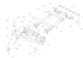
ЕТВ-6000000242, Рама левая
