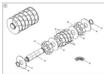
ETB-0000007900, Дозирующий ролик 210 см³
