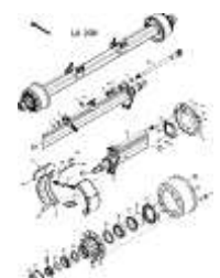
ЕТВ-0000003231, Оси (2)
