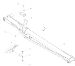
ЕТВ-6000000248, Рычаг
