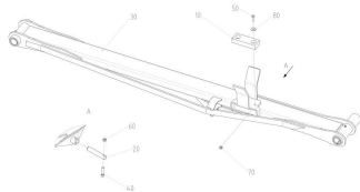
ЕТВ-6000000251, Рычаг
