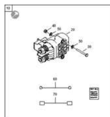
ETB-0000007496, Реле обмена (для NM067)
