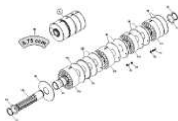
ETB-0000007608, Дозирующий ролик 3,75 см³
