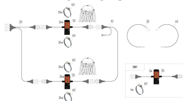
ЕТВ-6000000228, 66500362 Система контроля высева семян для DMC 9000 и 12000 с 48 сошниками с СКИФ-28 в базе (опция) до 05.2025
