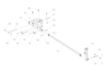
ЕТВ-6000000249, Тяга
