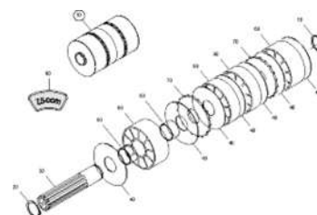
ETB-0000009075, Дозирующий ролик 7,5 куб.см
