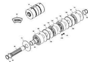
ETB-0000006887, Дозирующий ролик 7,5 куб.см с 8.2022
