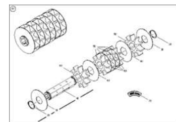
ETB-0000007897, Дозирующий ролик 600 куб.см
