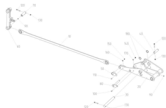
ЕТВ-6000000252, Тяга
