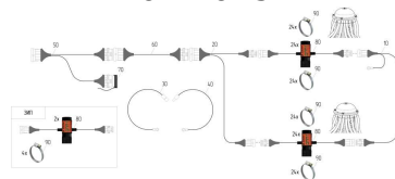
ЕТВ-6000000128 66500687 Базовый комплект электроники СКИФ-38 с 07.2025
