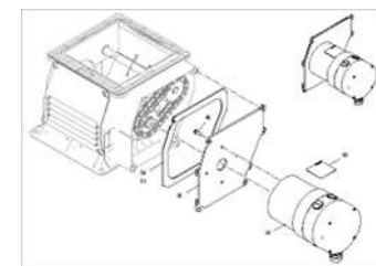
ЕТВ-0000007182, Подмножество электроприводов
